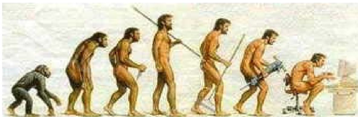
Homo erectocorvus
